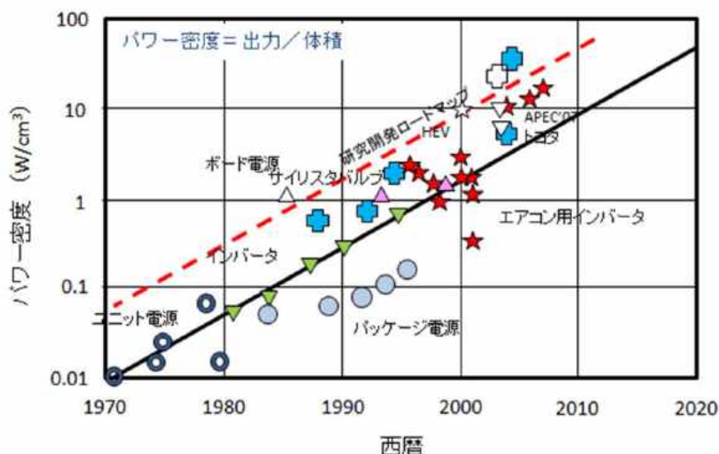
図付 1-3 電力変換器のパワー密度上昇 [5]
