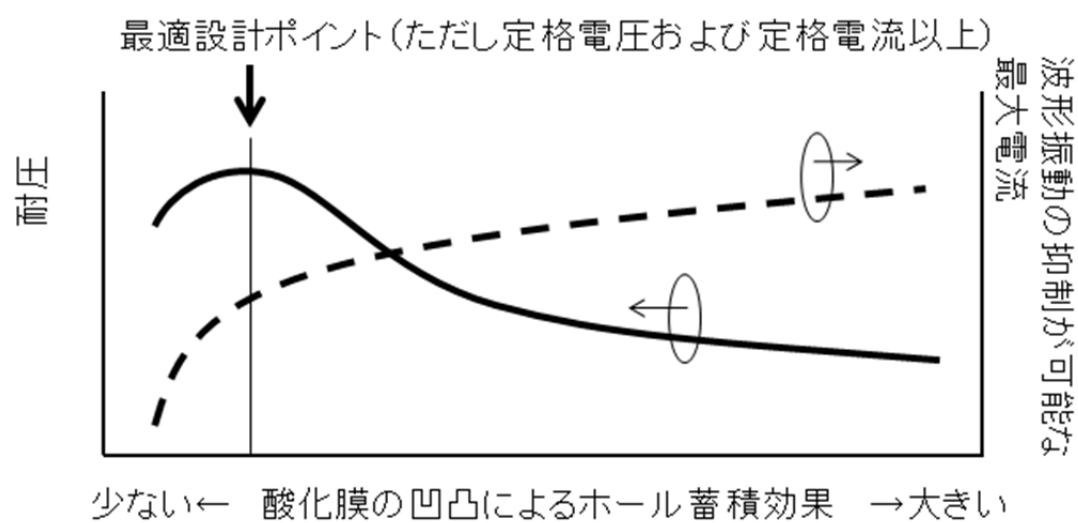
図 62 凹凸 SOI 構造を用いた PiN ダイオードの設計ガイドライン
