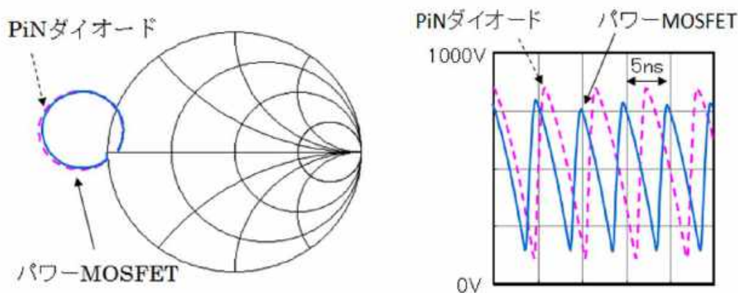
図 50 パワーMOSFET と PiN ダイオードの S パラとアバランシェ振動
